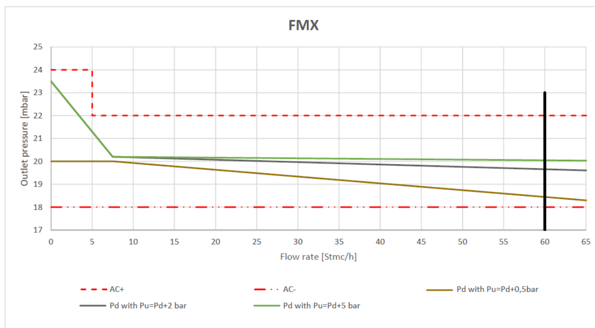
12. Charakterystyka przepływów reduktorów FMX
